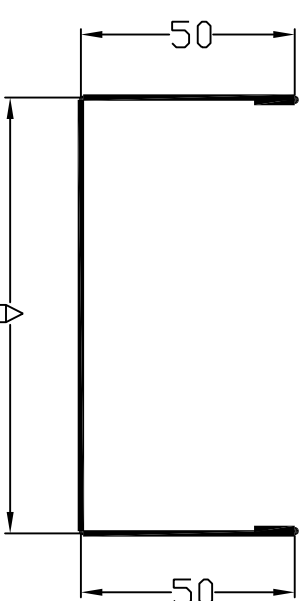
Perfil U dinteles
